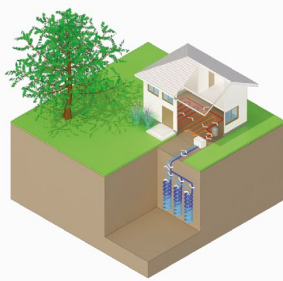
Pompe à chaleur sur corbeilles géothermiques
